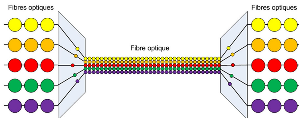
WDM ใช้ในการรับ - ส่ง สัญญาณแสงผ่านใยแก้วนำแสง (Fiber Optic)
