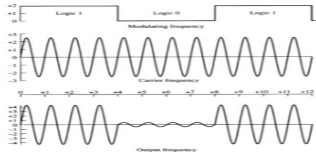
วิธีการแปลง Amplitude เรียกว่า Amplitude Shift Keying
